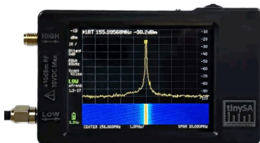
The tinySA
